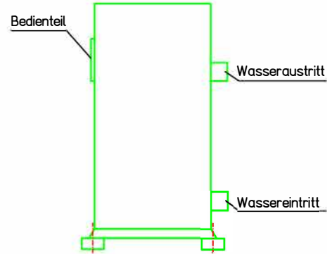
Vorderansicht
