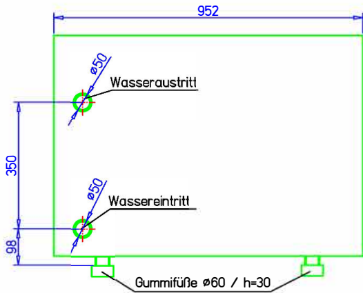
Seitenansicht von rechts
